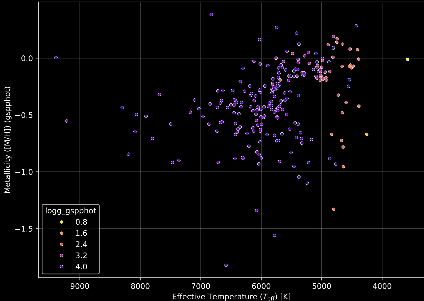
GALAH DR4 Field: [3141] Stellar Population Parameters (n= 237)
