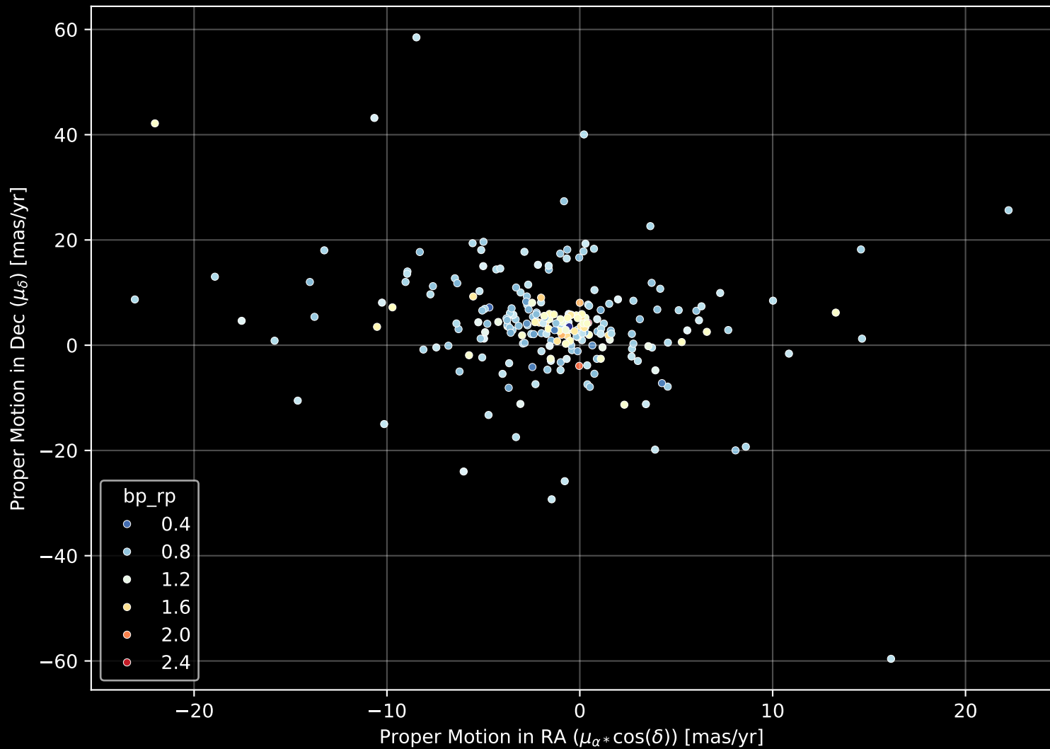
GALAH DR4 Field: [3141] Proper Motion Diagram (n= 237)
