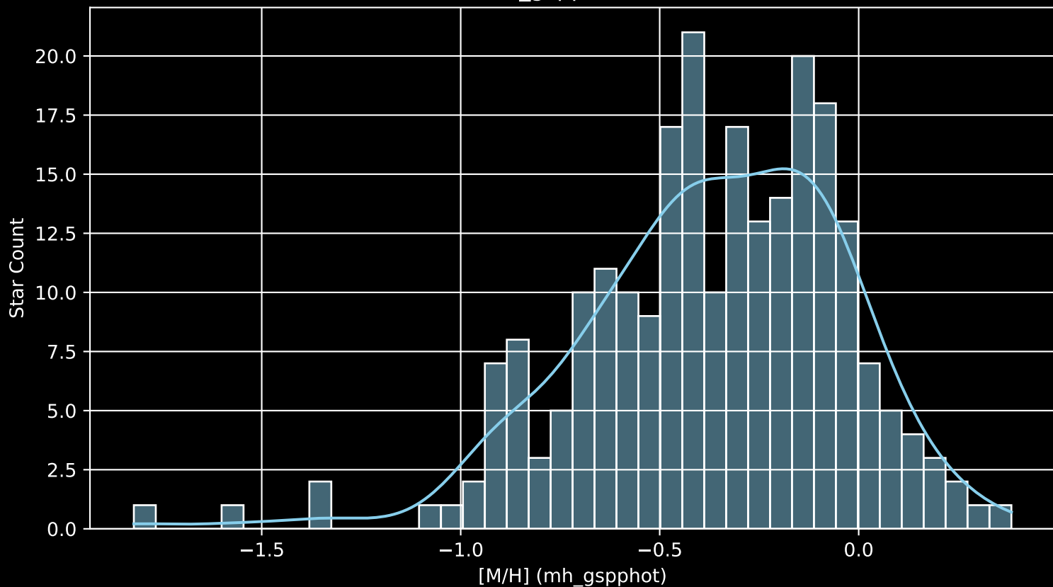
GALAH DR4 Field: [3141] [M/H] (mh_gspphot) (n= 237)
