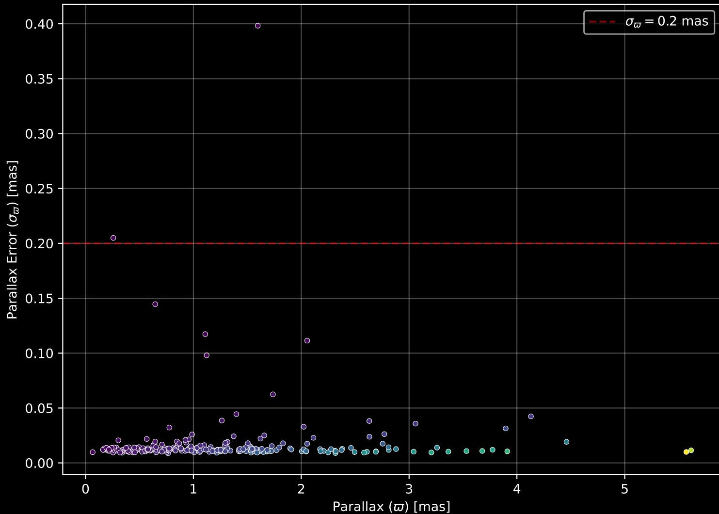
GALAH DR4 Field: [3141] Parallax Quality (n= 237)
