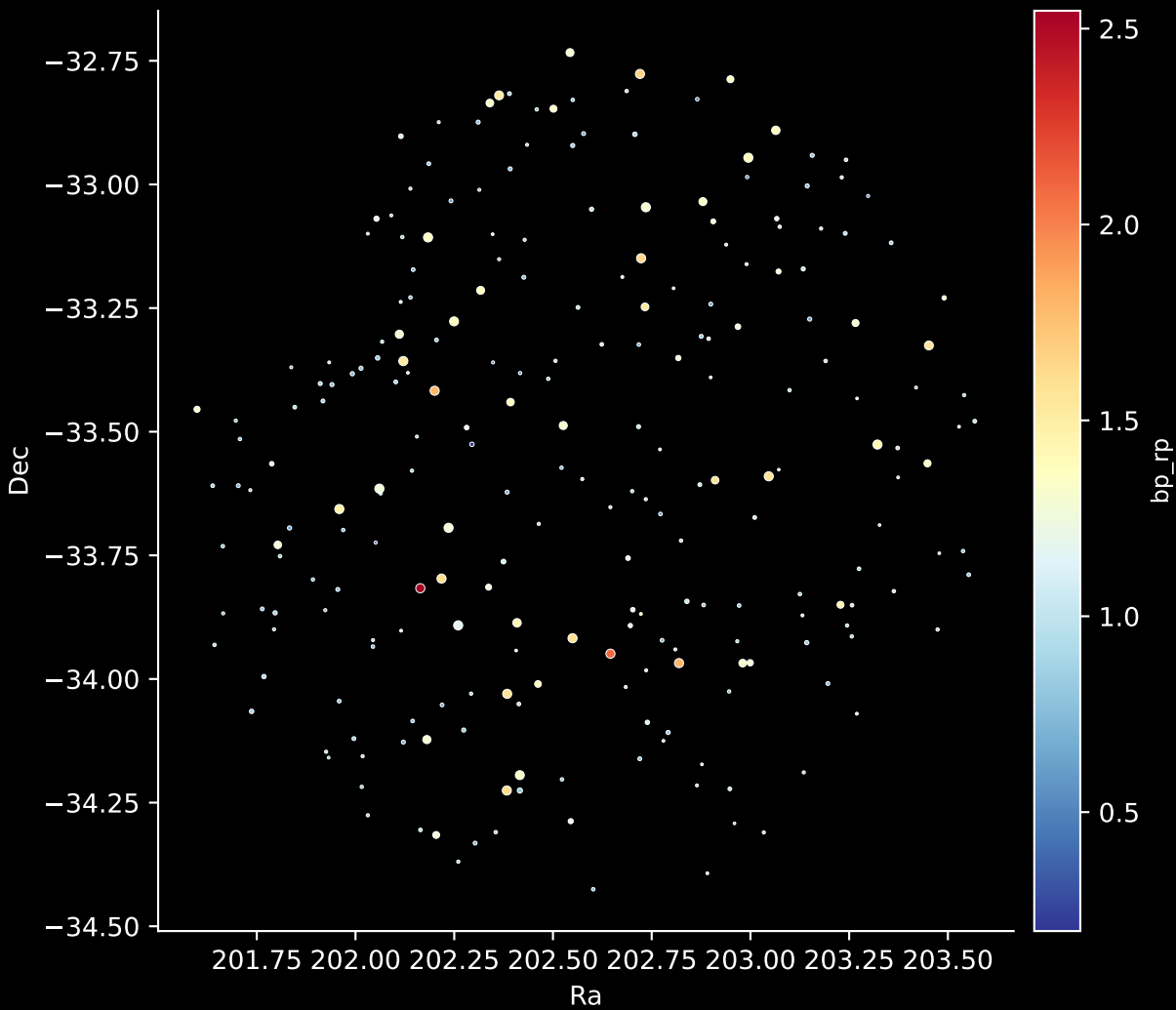
GALAH DR4 Field: [3141] Stars: 237
